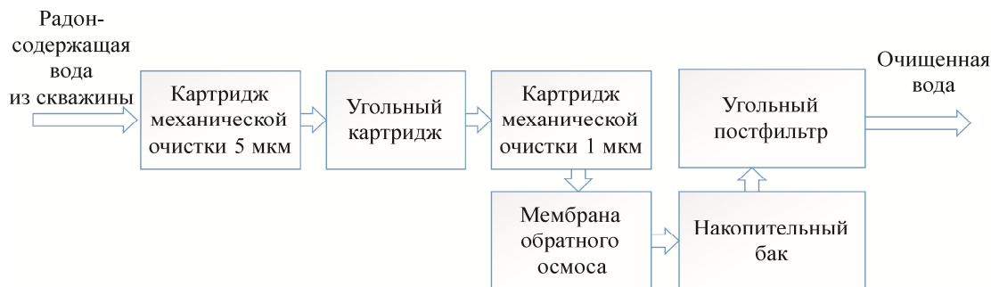
Рис. 2. Блок-схема очистки природной воды от радона мембраной фильтрацией
