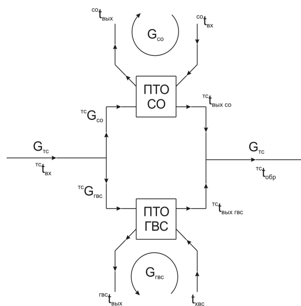
Рис. 1. Одноступенчатая параллельная схема
