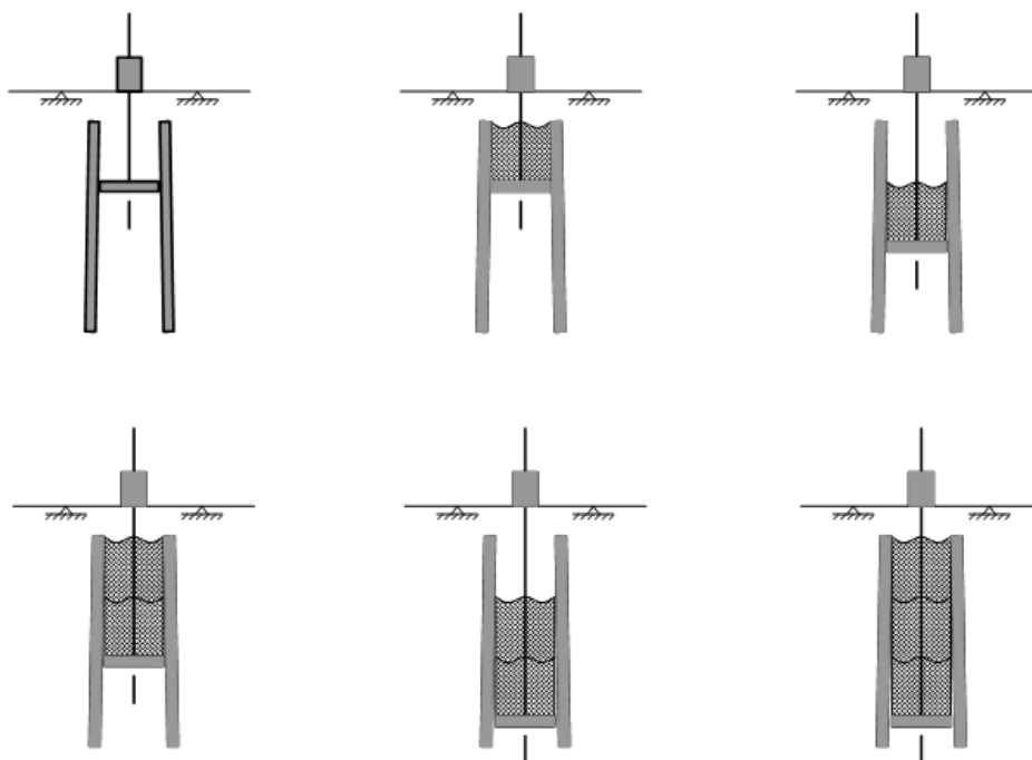
Принципиальная схема бетонирования методом опускающегося бетона по этапам
