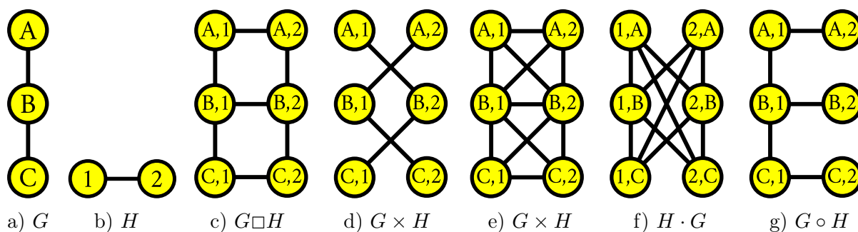
Рис. 2. Различные произведения графов
