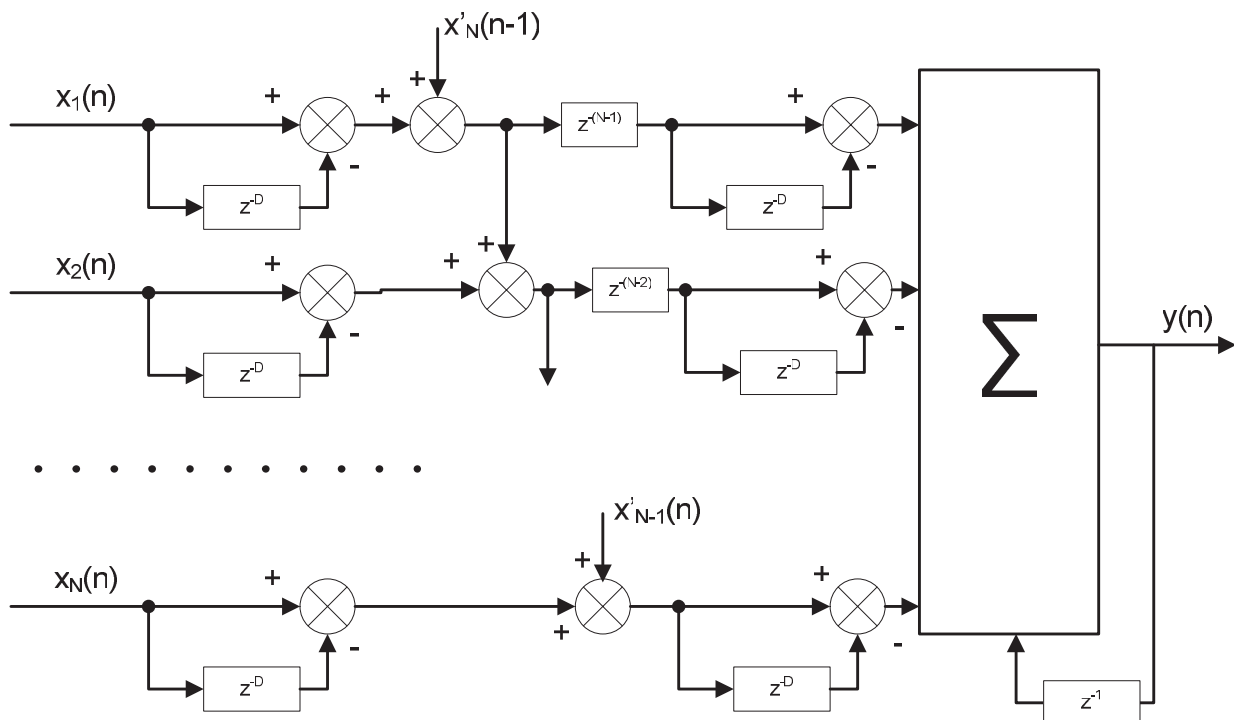
Рис. 5. Полифазный СИС-фильтр 2-го порядка
