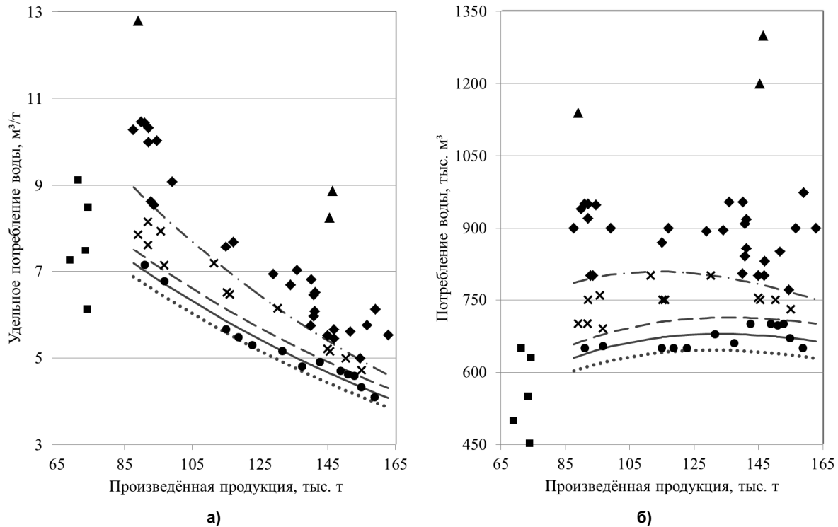
Рис. 2. Пример построения норм потребления технической воды
