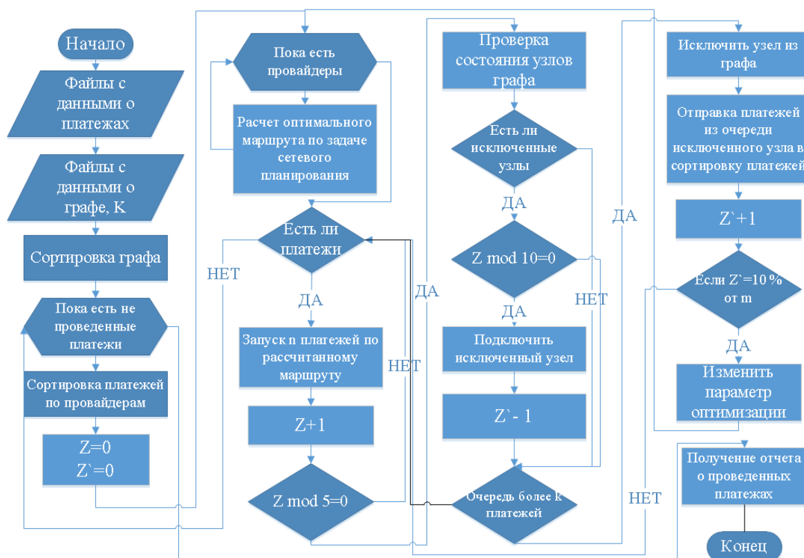
Алгоритм работы модуля проведения платежей: Z – количество итераций, Z' – количество исключенных узлов, m – общее количество узлов сети посредников, k – пороговое число очереди у посредника
