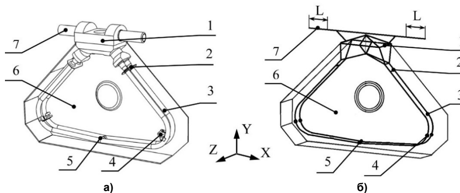
Рис. 3. Схема (а) и расчетная модель (б) системы «расходомер – трубопроводы»: 1 – основание (BEAM188); 2 – перемычки (BEAM188); 3 – трубки (BEAM188); 4 – измерительные катушки (MASS21); 5 – задающая катушка (MASS21); 6 – корпус (SHELL181); 7 – трубопроводы (BEAM188)
