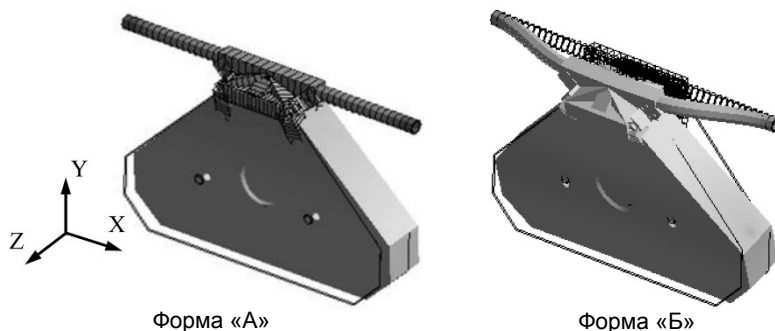
Рис. 5. Собственные формы колебаний системы «расходомер – трубопроводы», соответствующие частоты которых зависят от длин трубопроводов и расположены вблизи «рабочей» частоты
