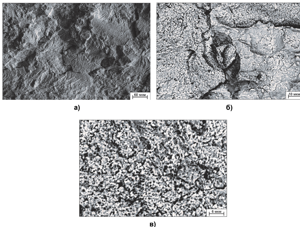
Рис. 2. Изломы образцов из алюминидов никеля, полученного спеканием методом SPS с различным содержанием циркония, после испытаний на трехточечный изгиб: а – 0,1 масс.%, б – 1 масс.% и в – 5 масс.%
