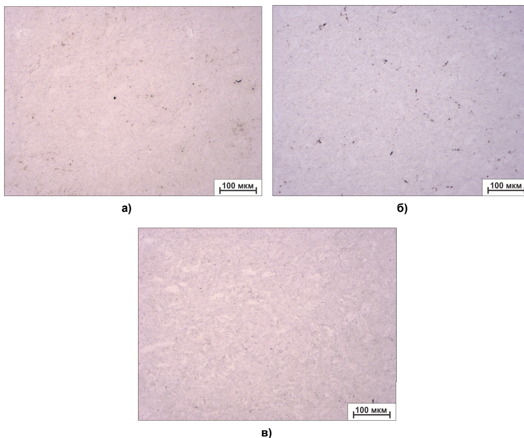
Рис. 1. Структура спеченного материала на основе алюминида никеля, зафиксированная на оптическом микроскопе, с добавлением 0,1 (а), 1 (б) и 5 (в) масс.% циркония
