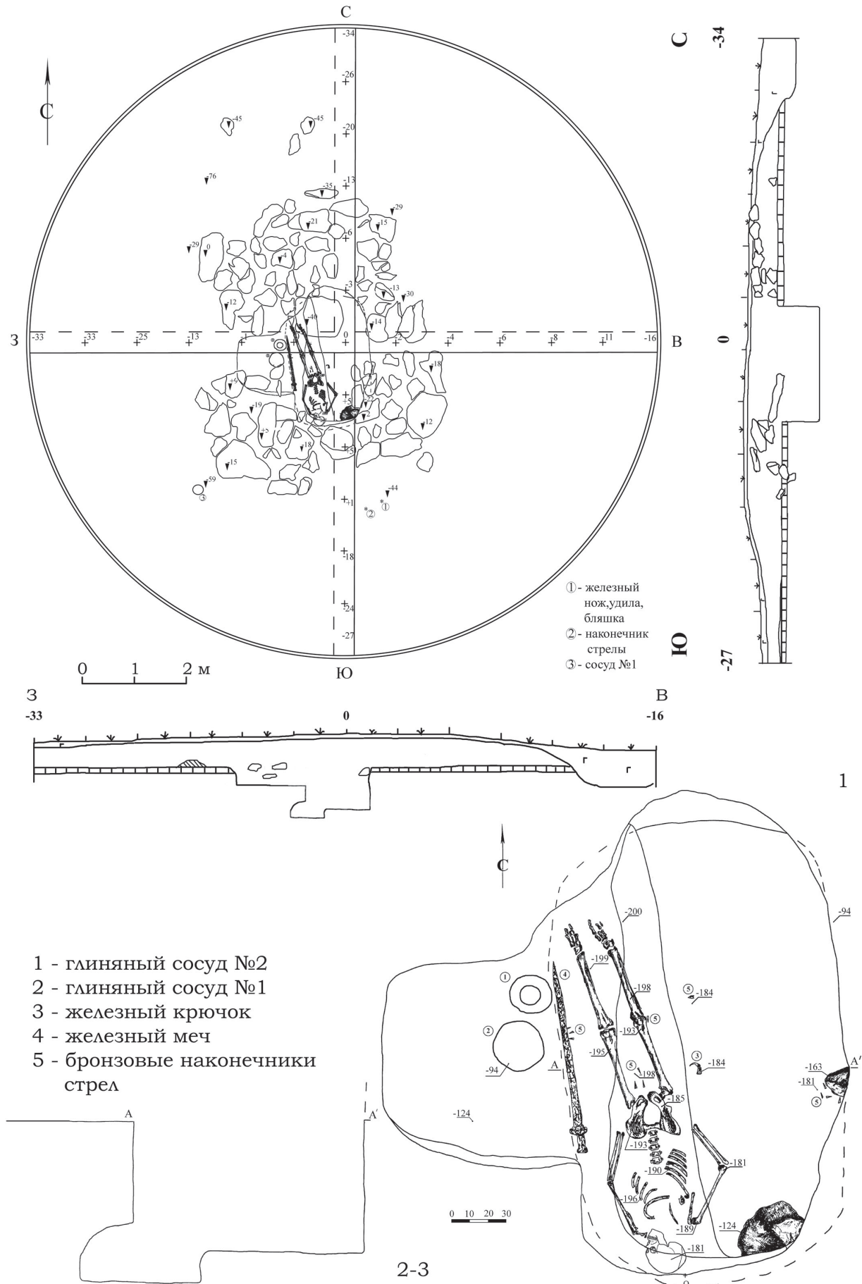
Рис. 2. Могильник Ушкатинский I, курган 8. 1 — план и разрезы кургана. 2-3 — план и разрез погребения 2
