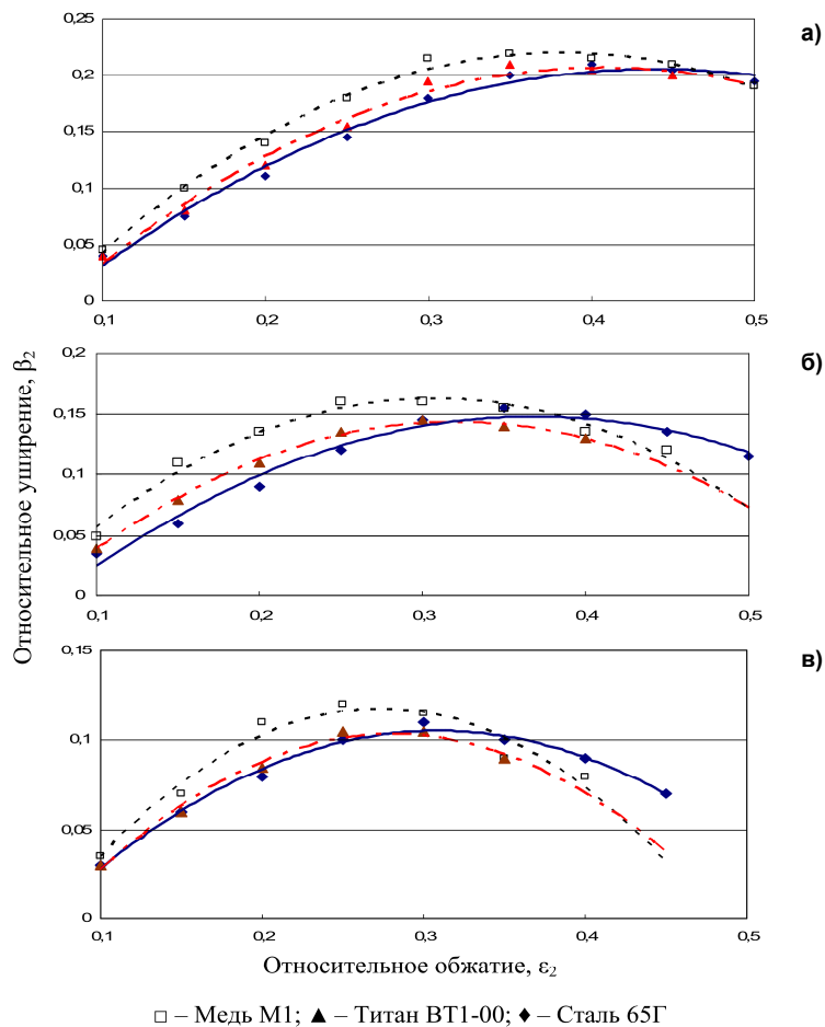
Рис. 2. Зависимость относительного уширения \beta_2 от относительного обжатия \varepsilon_2 для второй пары роликов при величине относительного обжатия в первой паре роликов: \varepsilon_1 = 0,20 (а); \varepsilon_1 = 0,25 (б); \varepsilon_1 = 0,30 (в)
