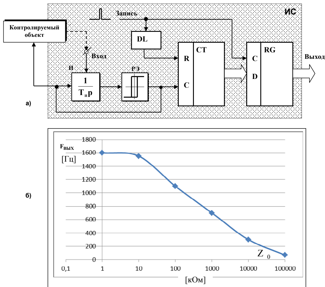
Рис. 1. Обобщенная структурная схема (а) и статическая характеристика (б) аналого-цифрового индикатора значения комплексного сопротивления изоляции
