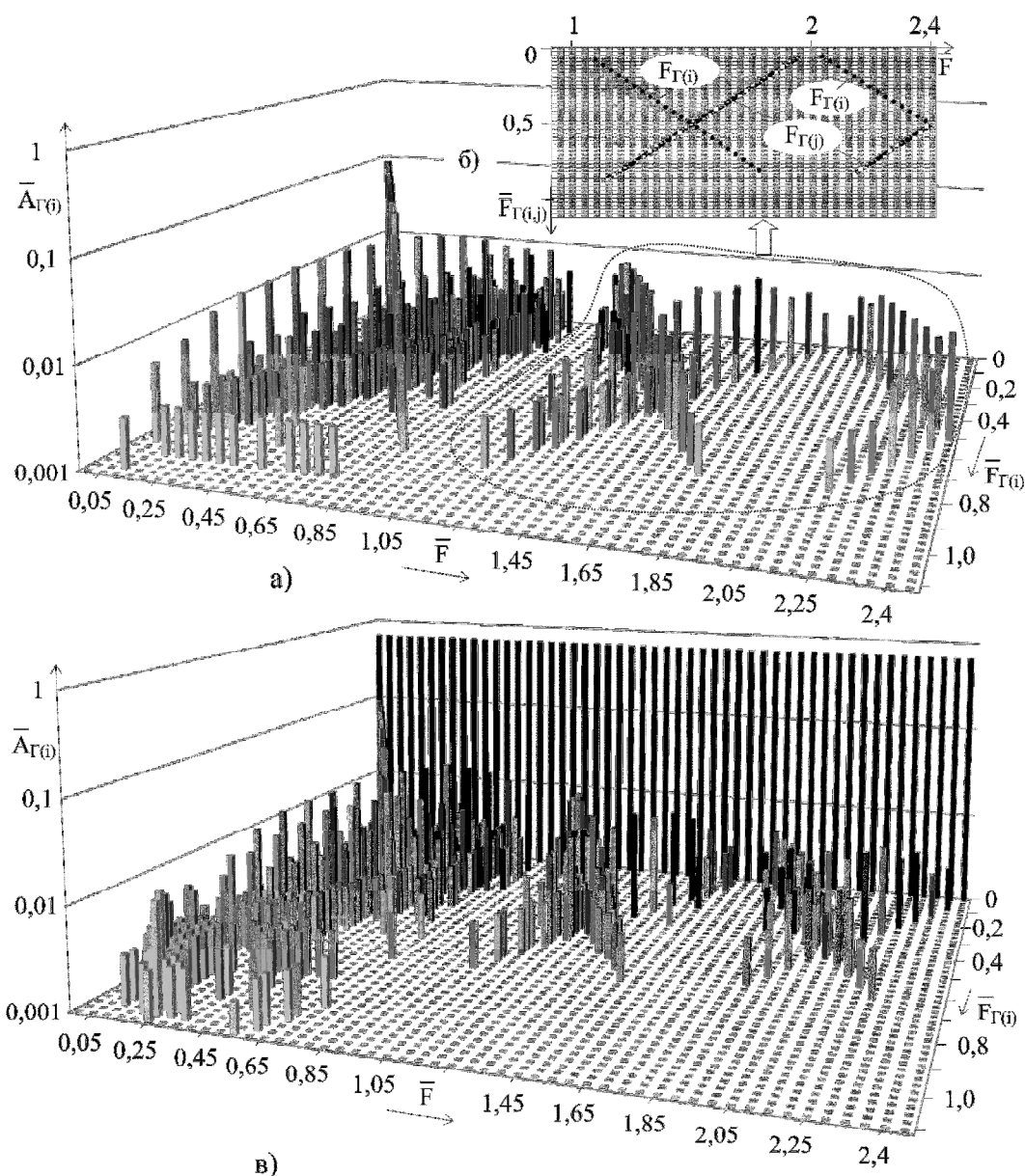
Рис. 4. Пространство динамического спектрального состояния МРП \bar{A}_{Г(t)} = f(\bar{F}, \bar{F}_{Г(t,i)}, \bar{A}_- = 0,1) при \bar{X}_{вх} = 0 (а), \bar{X}_{вх} = 0,8 (в) и проекция его фрагмента на плоскость переменных (\bar{F}, \bar{F}_{Г(t,i)}) (б)
