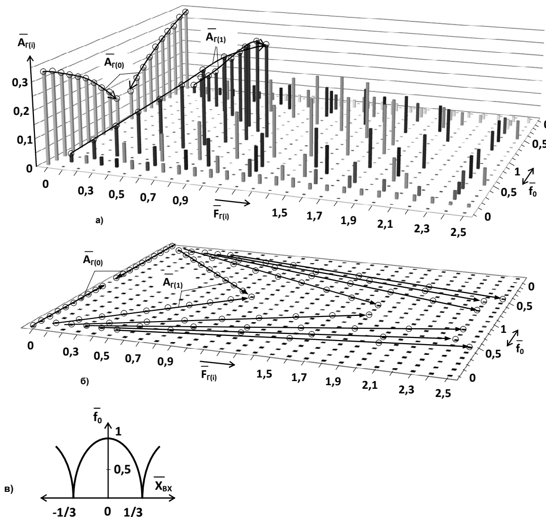
Рис. 3. Пространство спектрального состояния МРП \bar{A}_{\Gamma(i)} = f(\bar{F}_{\Gamma(i)}, \bar{f}_0) (а), его проекция на плоскость переменных (\bar{F}_{\Gamma(i)}, \bar{f}_0) (б) и модуляционная характеристика \bar{f}_0 = f(\bar{X}_{ВХ}) (в) для первой модуляционной зоны ( -1/3 < \bar{X}_{ВХ} < 1/3 )
