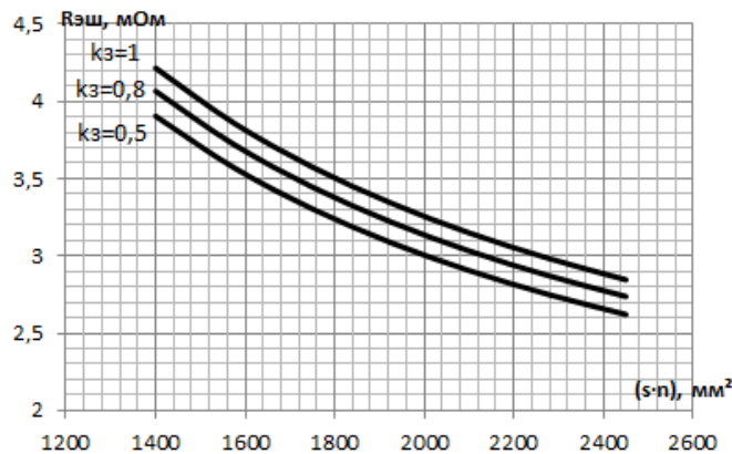
Рис. 5. Номограммы эквивалентного сопротивления шинпровода I_n = 250 \text{ А}, l_{\text{ср}} = 50 \text{ м}, \theta_0 = 35 \text{ °С}
